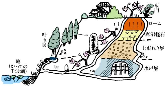
偕楽園南側斜面にみえる上市台地の断面
